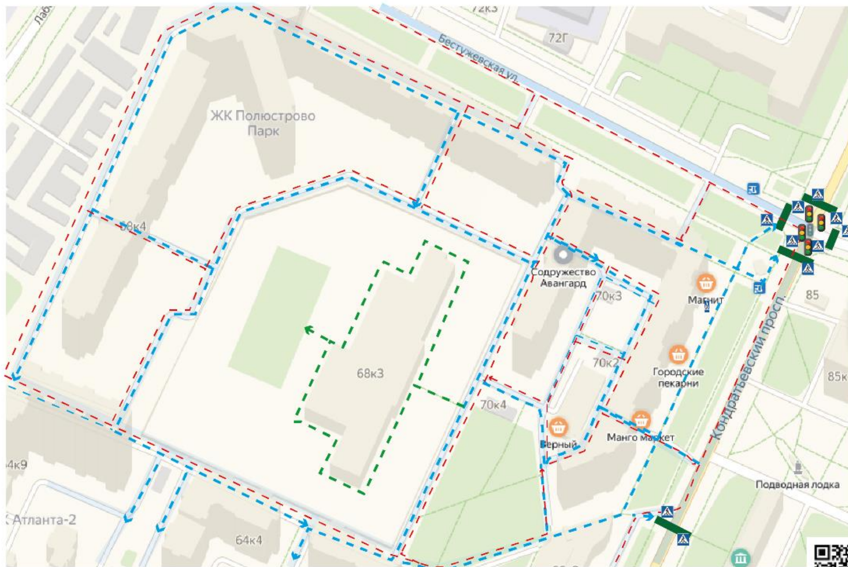
Схема организации дорожного движения в непосредственной близости от образовательного учреждения с размещением соответствующих технических средств, маршруты движения детей и расположения парковочных мест
